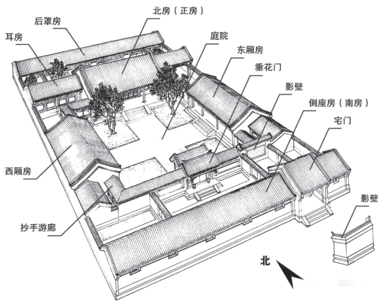
图3 四合院的结构图
